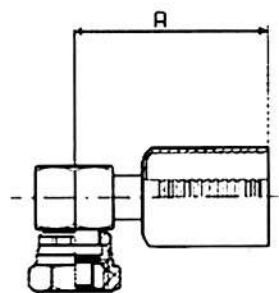
FITTINGS FOR STANDARD HOSE RACCORDI CON CAMPANA SEZIONE STANDARD
