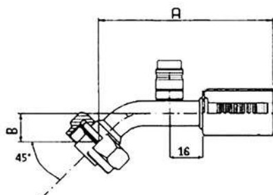
FITTINGS FOR STANDARD HOSE RACCORDI CON CAMPANA SEZIONE STANDARD
