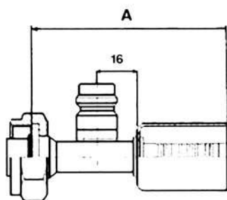
FITTINGS FOR STANDARD HOSE RACCORDI CON CAMPANA SEZIONE STANDARD
