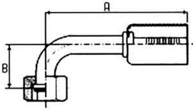
FITTINGS FOR STANDARD HOSE RACCORDI CON CAMPANA SEZIONE STANDARD
