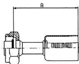
FITTINGS FOR STANDARD HOSE RACCORDI CON CAMPANA SEZIONE STANDARD
