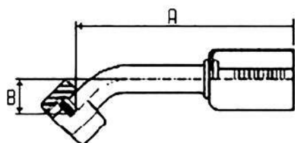
FITTINGS FOR STANDARD HOSE RACCORDI CON CAMPANA SEZIONE STANDARD
