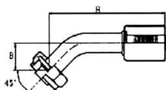
FITTINGS FOR STANDARD HOSE RACCORDI CON CAMPANA SEZIONE STANDARD
