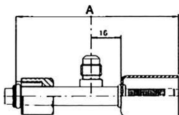
FITTINGS FOR STANDARD HOSE RACCORDI CON CAMPANA SEZIONE STANDARD
