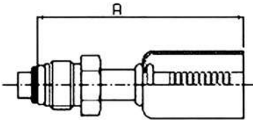
FITTINGS FOR STANDARD HOSE RACCORDI CON CAMPANA SEZIONE STANDARD
