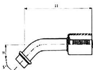
FITTINGS FOR STANDARD HOSE RACCORDI CON CAMPANA SEZIONE STANDARD
