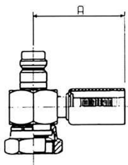
FITTINGS FOR STANDARD HOSE RACCORDI CON CAMPANA SEZIONE STANDARD
